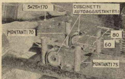
6 - La sistemazione del motore dipende dal tipo adottato. Nel prototipo è stato usato il supporto qui raffigurato: quattro montanti saldati al telaio
