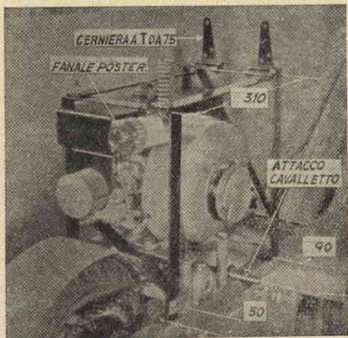
11 - Notate la sistemazione del sedile al di sopra del motore, incernierato anteriormente per un più facile accesso al motore stesso. Di fianco al motore trova posto il serbatoio per il carburante. Dietro è sistemato il fanalino posteriore. Come sedile consigliamo un cuscino di gomma piuma fissato su di una tavola di compensato.
