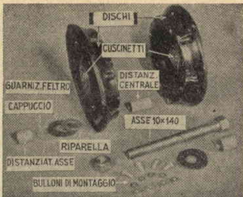
4 - Preparazione del mozzo della ruota - I cuscinetti sono a posto nei cerchioni. Il distanziatore centrale deve esser serrato contro gli anelli interni dei cuscinetti, la cui vite è prolungata da guarnizioni di feltro. Bulloni e dadi tengono unito il mozzo.
