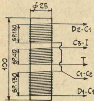
Fig. 2 BOBINA
