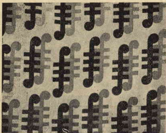
Bastano due colori per un effetto di prim'ordine
