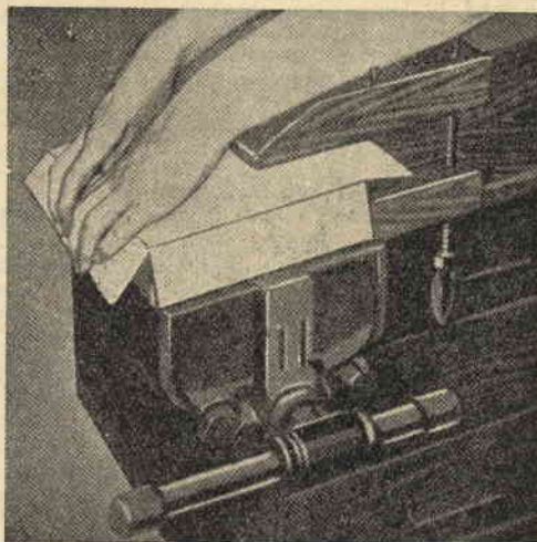
Fig. 4 - Come va piegata la lamiera
