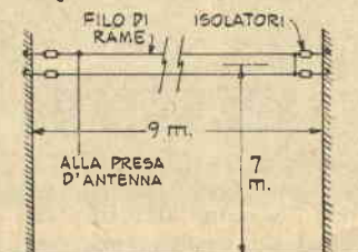
Fig. 3 ANTENNA
